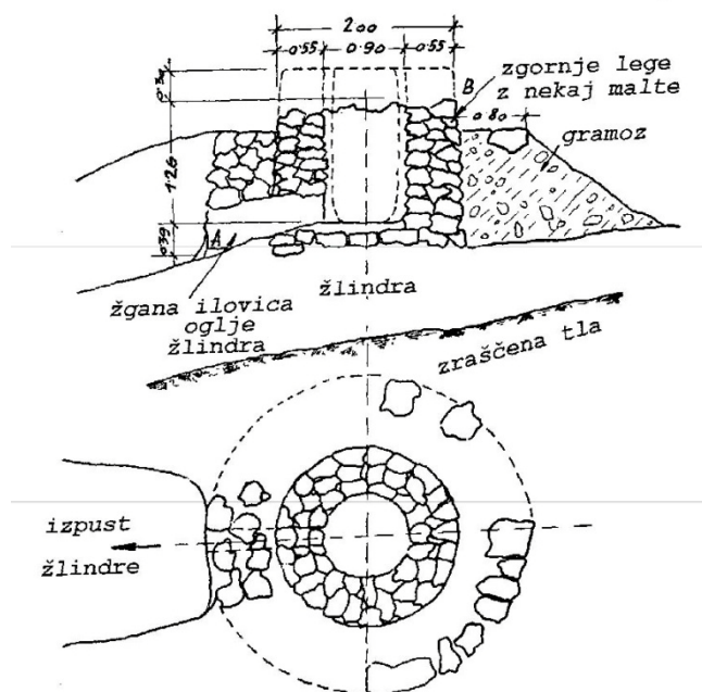
Rimskodobna kupolasta peč v Löllinga. 41
