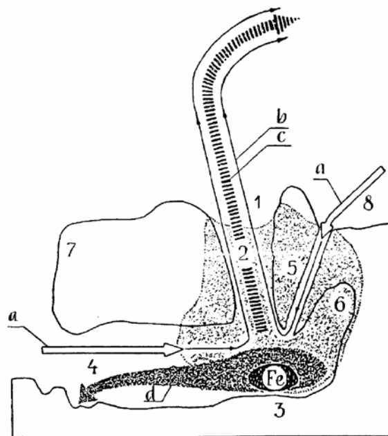
Slika 31. Češka staroslovanska topilna peč – Želechovice □B16,s.212,sl.56□
