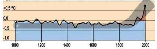
Temperaturabweichung Relativ zu 1980 - 1990 Der "hockey stick" des IPCC +1,0 +0,5 °C 0,0 -0,5 -1,0
