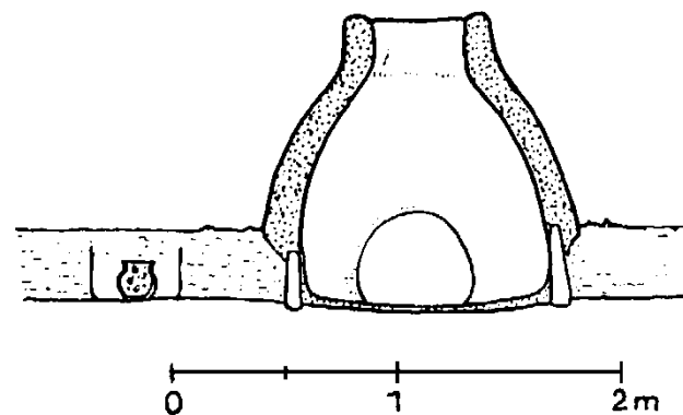
Latenska kupolasta železarska
