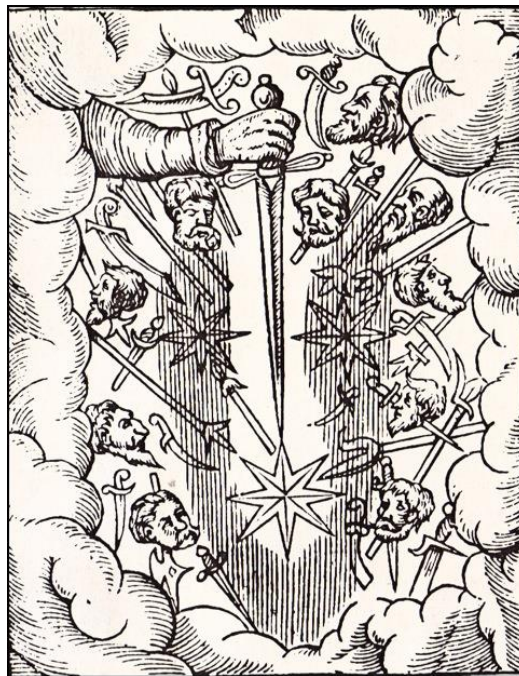
Velik komet iz leta 1527 – srednjeveška gravura pravzaprav prikazuje, kako so si komet predstavljali nekateri sodobniki.
